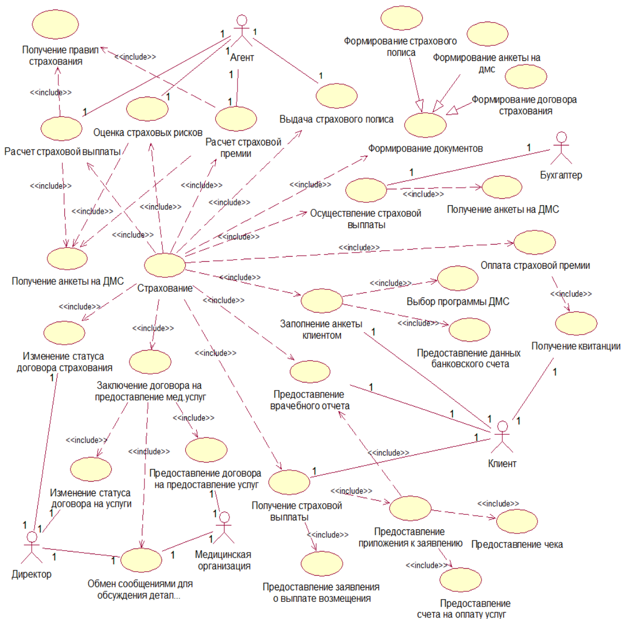
Рисунок 1 – Диаграмма вариантов использования процесса страхования
